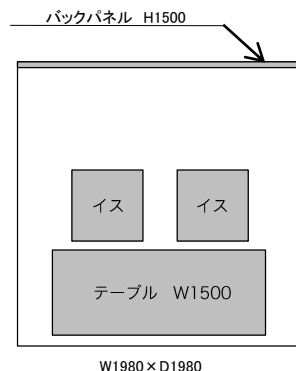
【平面図】
